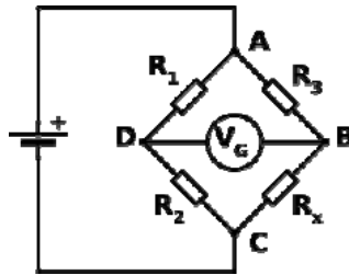
Şekil 2. R_x strain gage'li tipik Wheatstone köprü diyagramı
